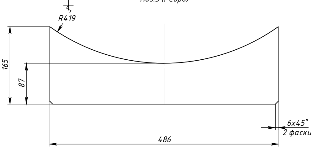
Поз.3 (Ребро)
